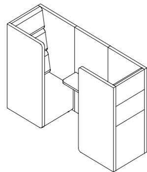
ALL14 W 2230 D 700 H 1500
