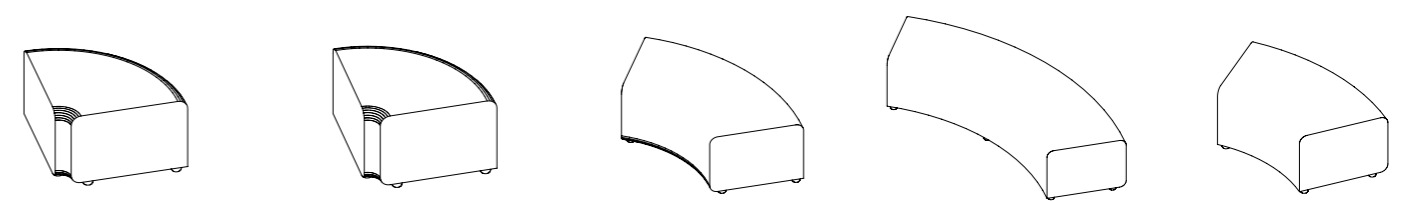
ALL19 90 DEG W 660 D 660 H 450 ALL20 90 DEG W 800 D 800 H 450 ALL21 60 DEG W 1180 D 595 H 450 ALL22 60 DEG W 2235 D 595 H 450 ALL23 45 DEG W 1175 D 595 H 450
