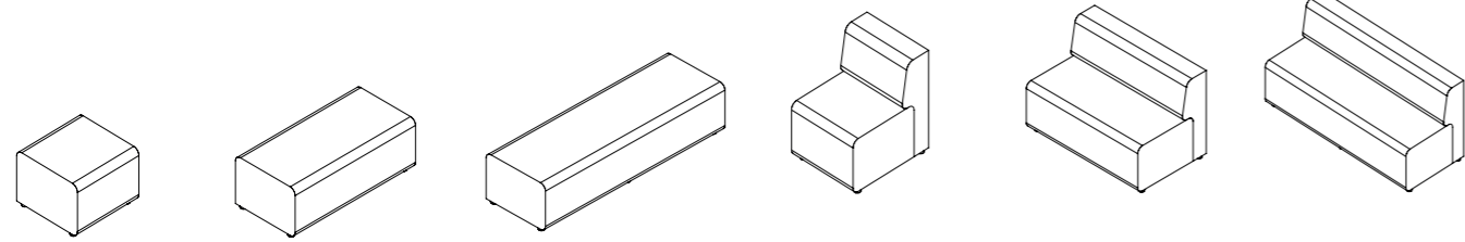
ALL01 ALL02 ALL03 ALL04 ALL05 ALL06 W 600 D 595 H 450 W 1200 D 595 H 450 W 1800 D 595 H 450 W 600 D 735 H 800 W 1200 D 735 H 800 W 1800 D 735 H 800
