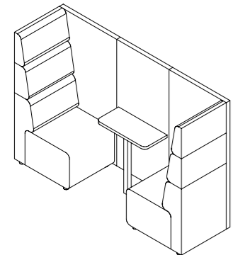
ALL13 W 2230 D 650 H 1500
