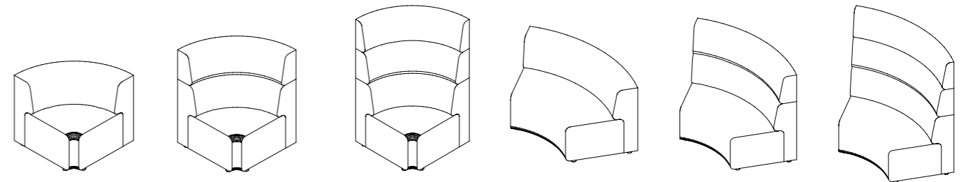
ALL24 90 DEG W 800 D 800 H 800 ALL25 90 DEG W 800 D 800 H 1150 ALL26 90 DEG W 800 D 800 H 1500 ALL27 60 DEG W 1500 D 735 H 800 ALL28 60 DEG W 1500 D 735 H 1150 ALL29 60 DEG W 1500 D 735 H 1500
