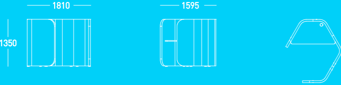
FLE HEX 001
